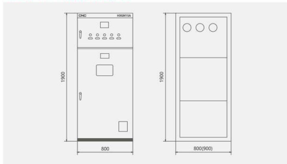
Габаритные и установочные размеры (мм)
