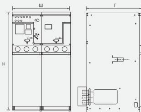
884×845×1550(Ш*Г*В) ячейка для подъема (перемещения)
