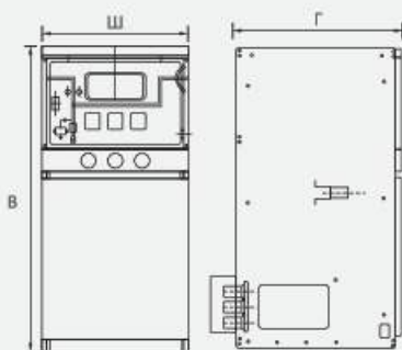
750×845×1550(Ш*Г*В) измерительная ячейка(стандартный тип)
