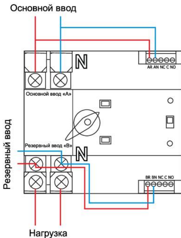
Схема подключения YCQ4E 100/4P
