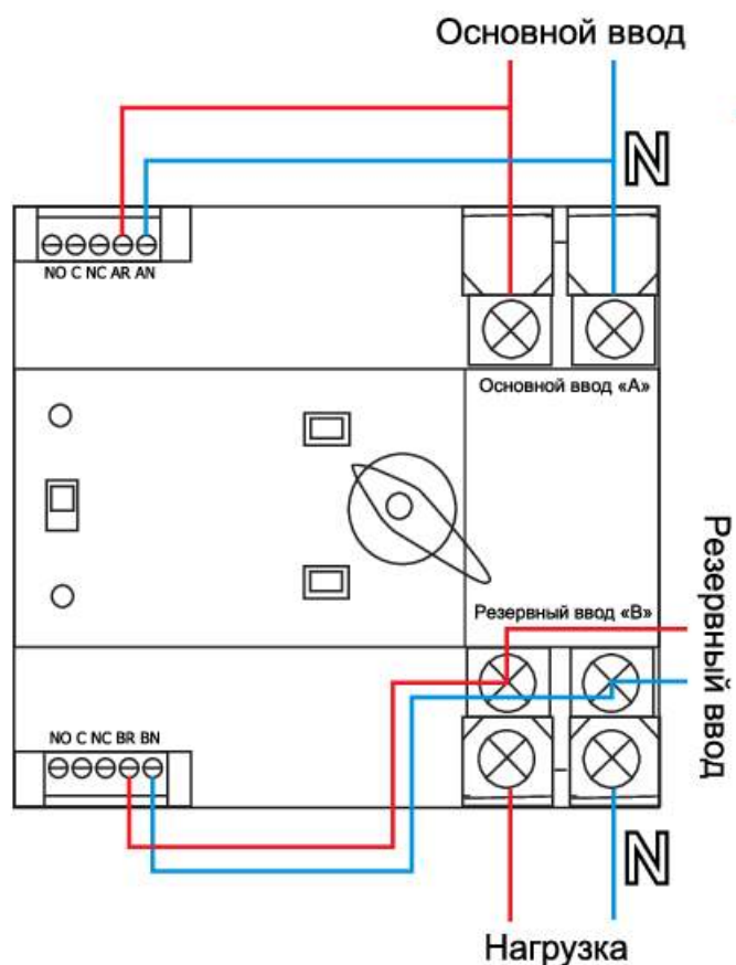
Схема подключения YCQ4R 100/4P
