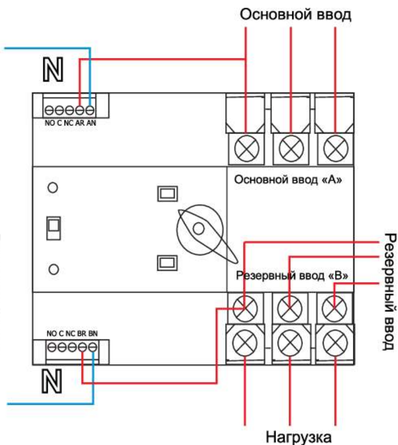
Схема подключения YCQ4R 100/4P
