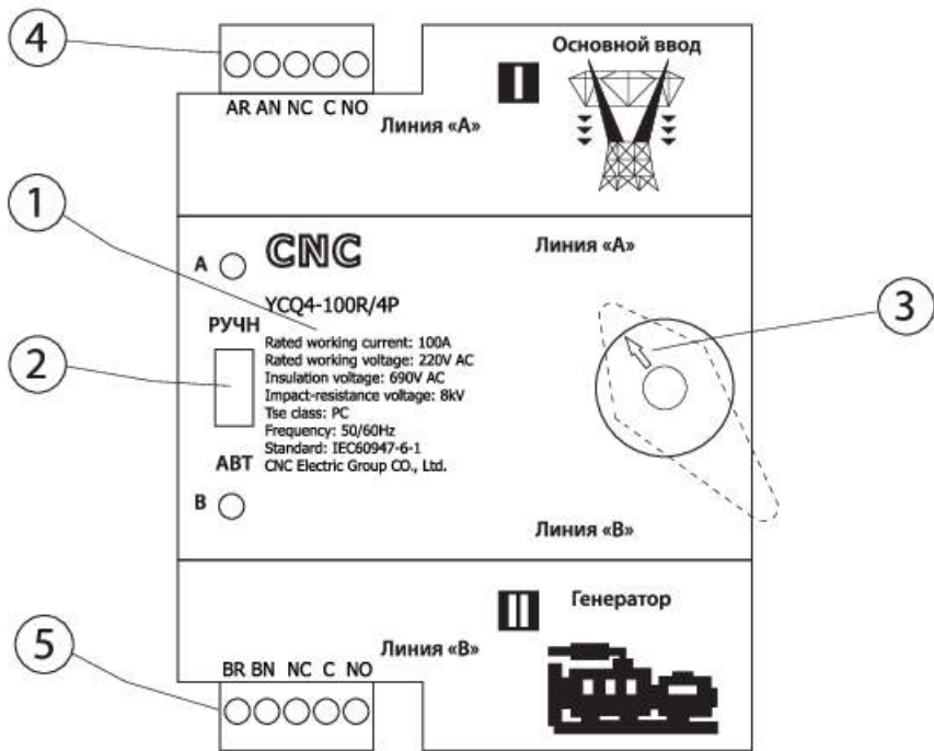
Панель управления контроллера
