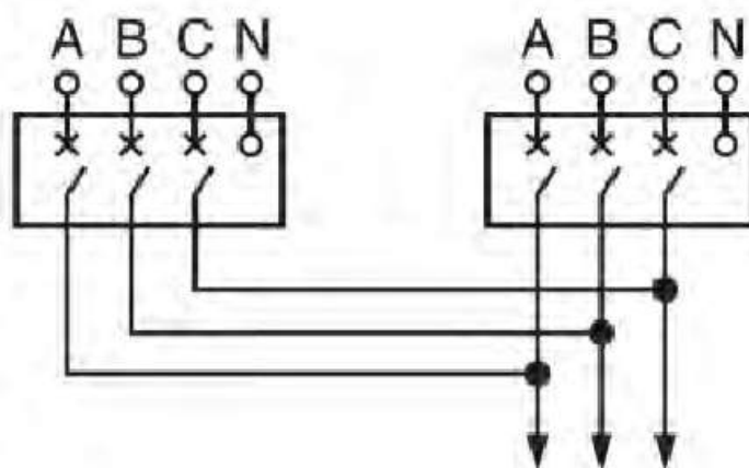
Схема подключения 3 полюсов
