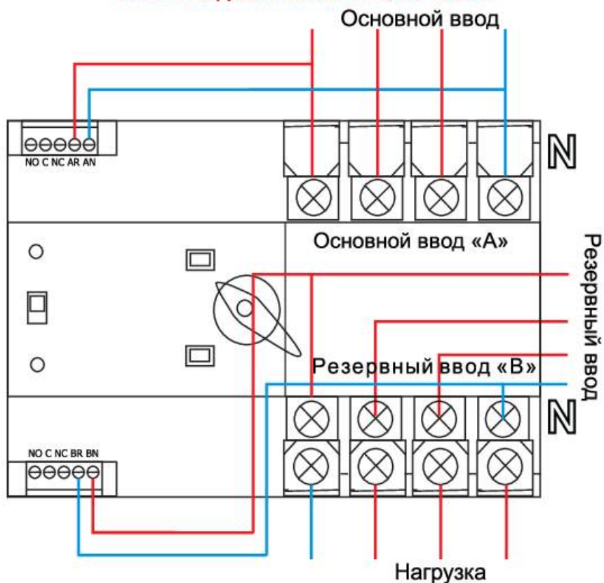
Схема подключения YCQ4R 100/4P
