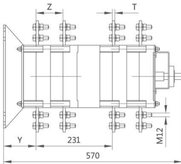
YCHGLZ1 2000-3200A с боковым управлением
