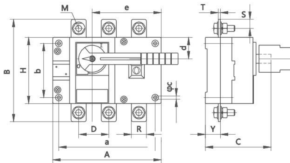
YCHGL(B) 160-630A прямого управления
