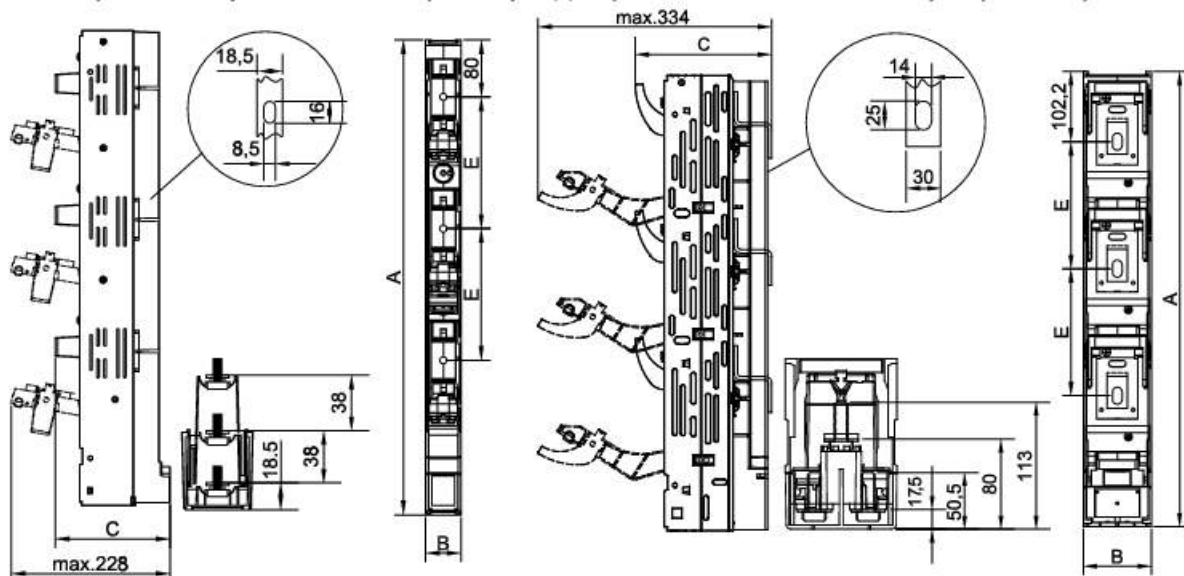
160 Габаритные и установочные размеры
