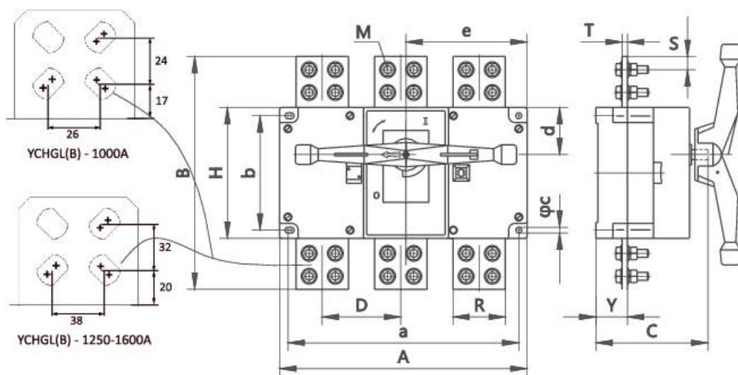
YCHGL(B) 1000-1600A прямого управления
