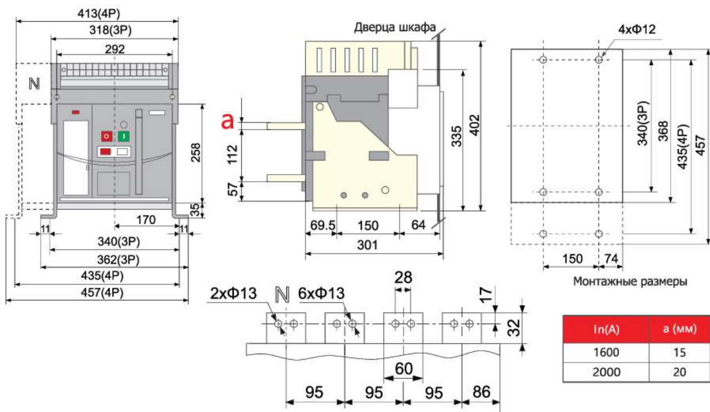
Габаритные и монтажные размеры автоматического выключателя стационарного типа YCW1 i - 2000A
