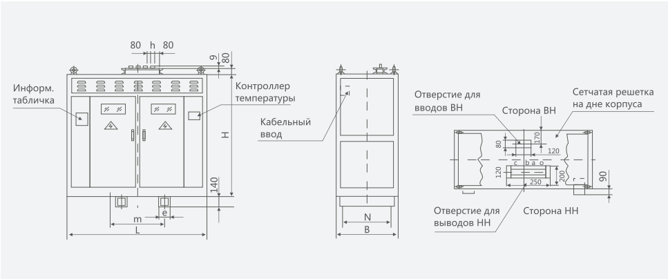
Присоединительные размеры вводов НН
