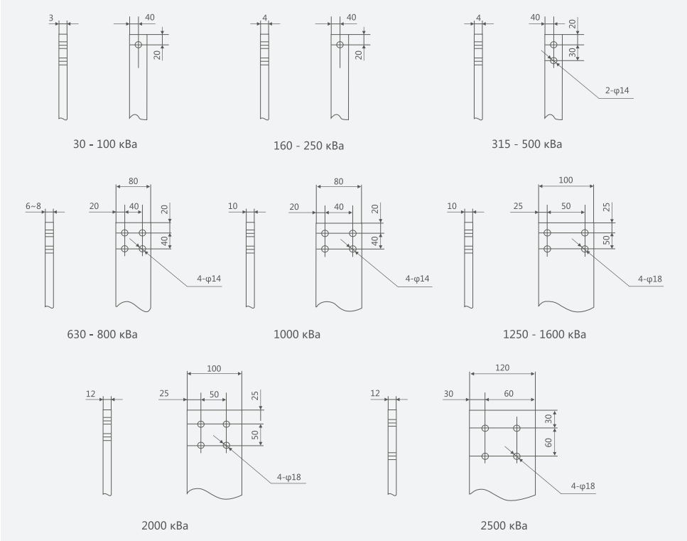
Присоединительные размеры вводов НН
